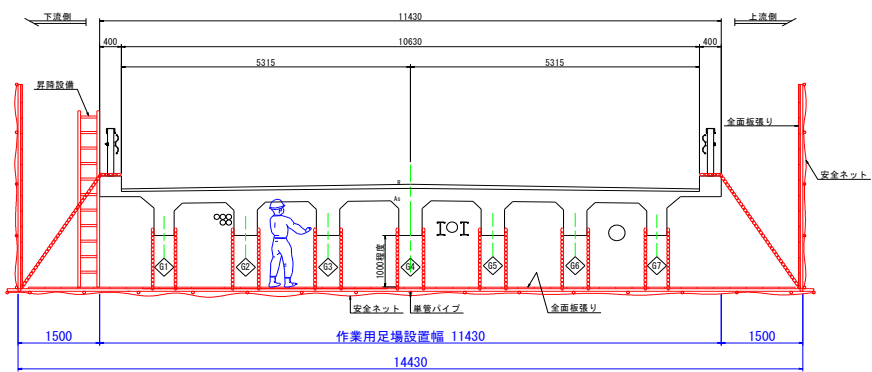
断面図
