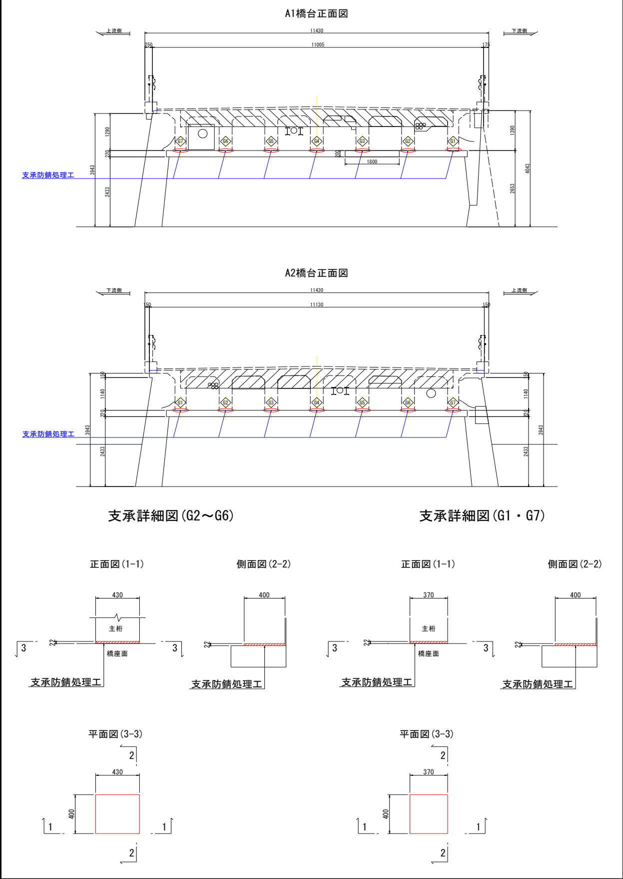
構造図
