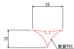
水切り詳細図(a部)
