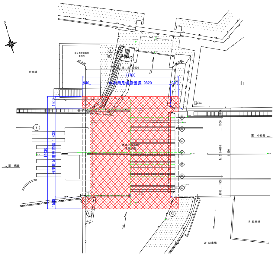
平面図
